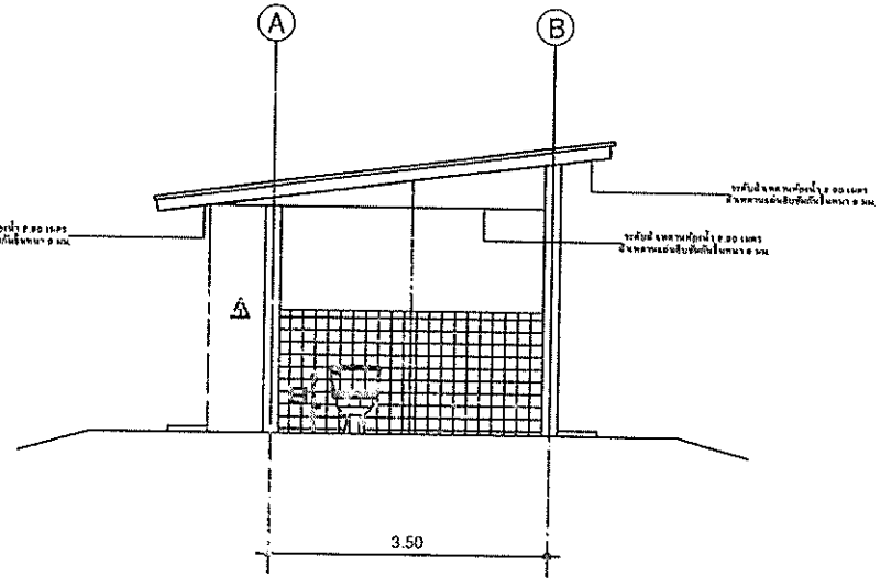
แบบแสดงรูปตัด B
