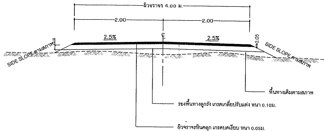
รูปตัดถนนลูกรัง NOT TO SCALE
