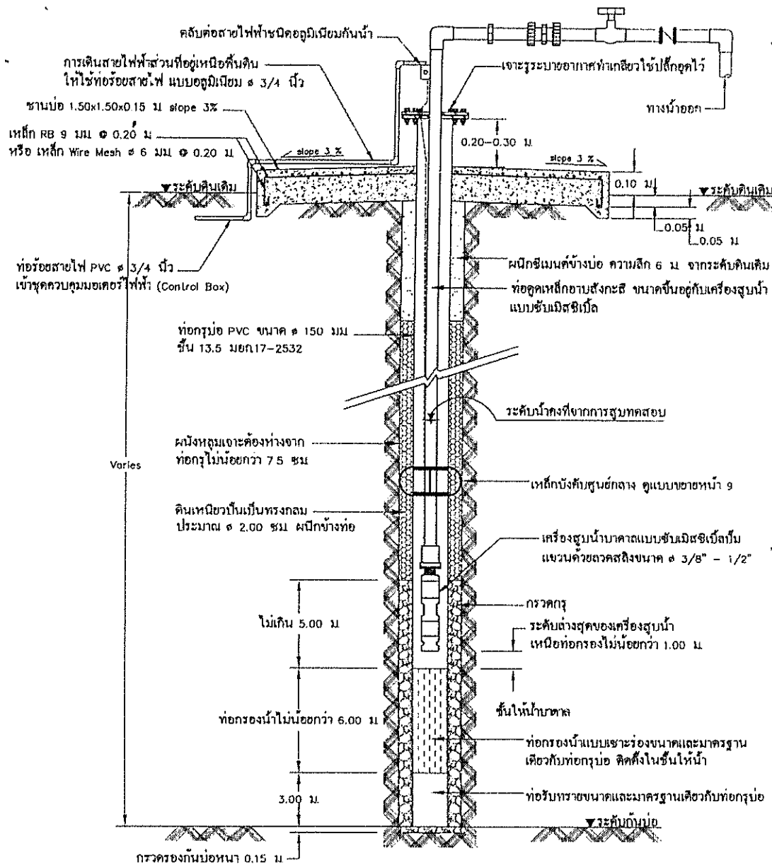
ภาพตัดบ่อน้ำบาดาลแบบกรวดรอบท่อ การติดตั้งเครื่องสูบน้ำบาดาล ระบบขับเคลื่อนสปีด Scale Not to Scale
