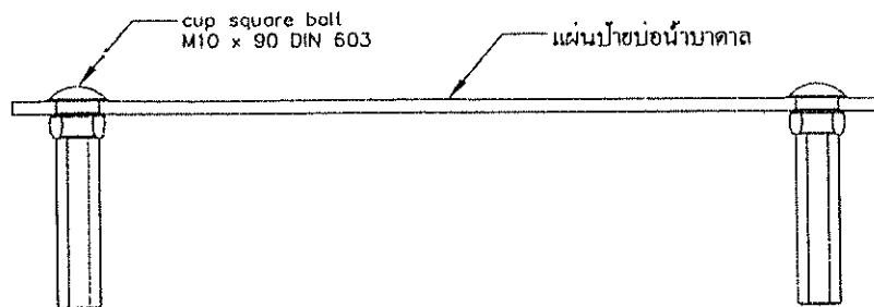
แผ่นป้ายสำหรับติดบนฐานคอนกรีตบ่อน้ำบาดาล
