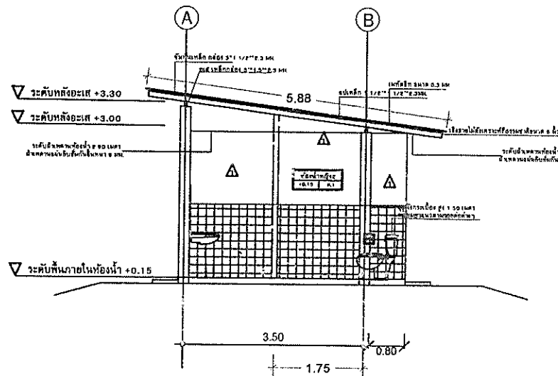
แบบแสดงรูปตัด A
