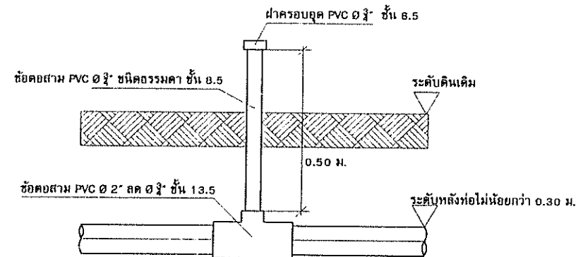
แบบสามทางแยกต่อขึ้น
