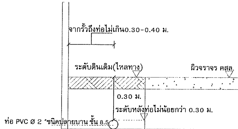
แบบวางท่อ
