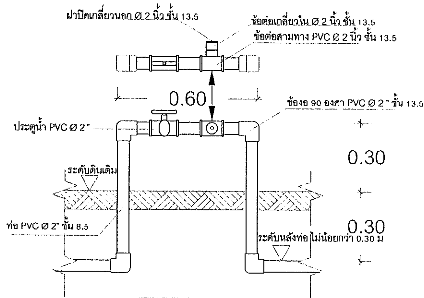
แบบขยาย 1
