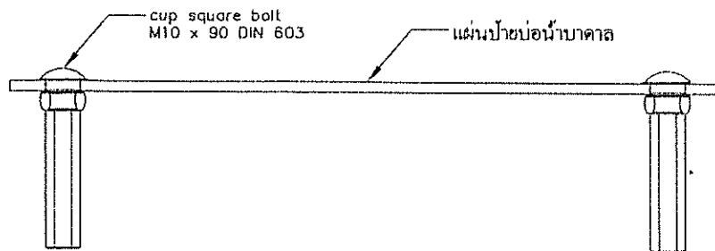
แผ่นป้ายสำหรับติดบนฐานคอนกรีตบ่อน้ำบาดาล Scale Not to Scale
