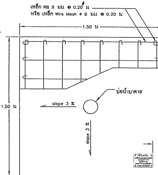
แบบฐานบ่อน้ำบาดาล Scale Not to Scale
