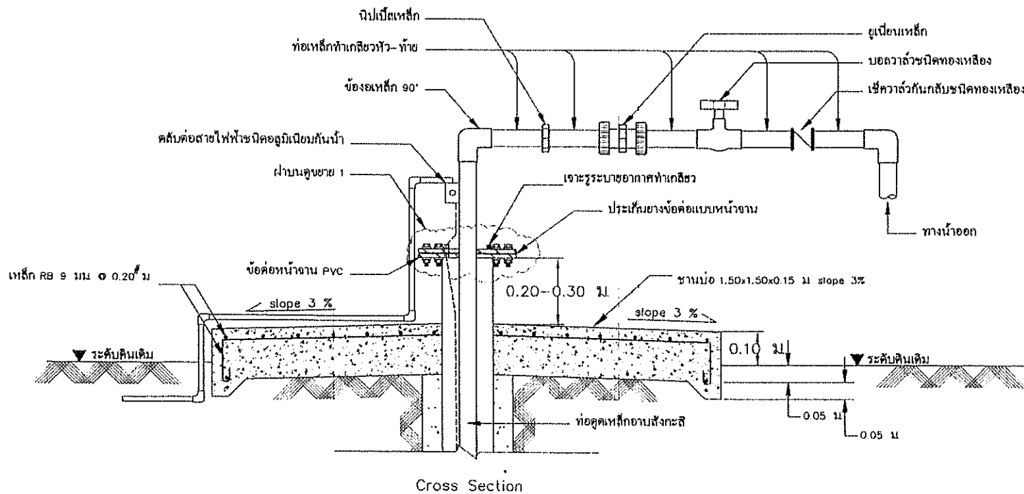
ขยาย 1 Scale Not to Scale
