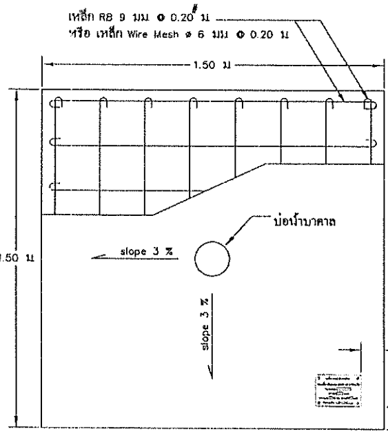
แบบขานบ่อน้ำบาดาล Scale Not to Scale
