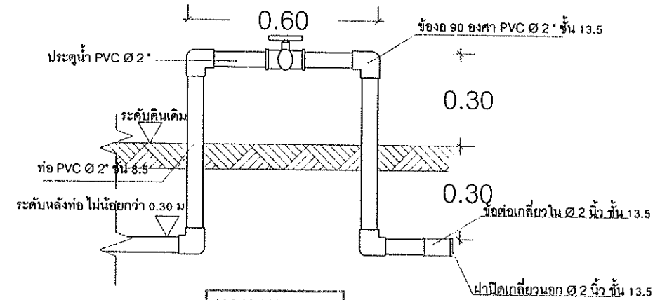
แบบขยาย 2
